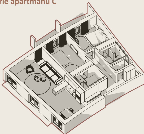
Axonometrie apartmánu C
